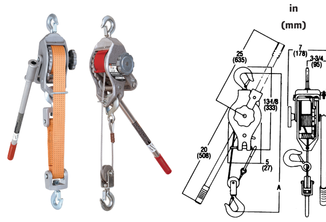
C-Series Pullers
