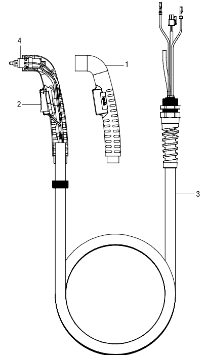
HP-25 Torch
