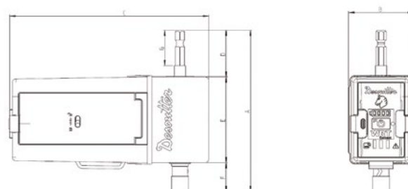
WRT4-Hex1/4, WRT10-Hex1/4, WRT20-Hex1/4
