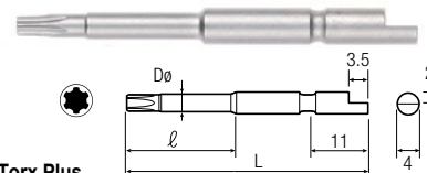
IP Dø I LENGTH L PART NO mm in mm in mm in 10 pcs 2IP 1.5 0.06 20 0.79 44 1.73 615 820 381 0 2IP 1.5 0.06 20 0.79 64 2.52 615 820 367 0 3IP 1.7 0.07 20 0.79 44 1.73 615 820 382 0 3IP 1.7 0.07 20 0.79 64 2.52 615 820 368 0 4IP 1.8 0.07 20 0.79 44 1.73 615 820 357 0 4IP 1.8 0.07 20 0.79 64 2.52 615 820 358 0 5IP 2.0 0.08 20 0.79 44 1.73 615 820 359 0 5IP 2.0 0.08 20 0.79 64 2.52 615 820 360 0 6IP 2.5 0.10 20 0.79 44 1.73 615 820 361 0 6IP 2.5 0.10 20 0.79 64 2.52 615 820 362 0 8IP 3.0 0.12 20 0.79 44 1.73 615 820 363 0 8IP 3.0 0.12 20 0.79 64 2.52 615 820 364 0 10IP 3.0 0.12 20 0.79 44 1.73 615 820 365 0 10IP 3.0 0.12 20 0.79 64 2.52 615 820 366 0
